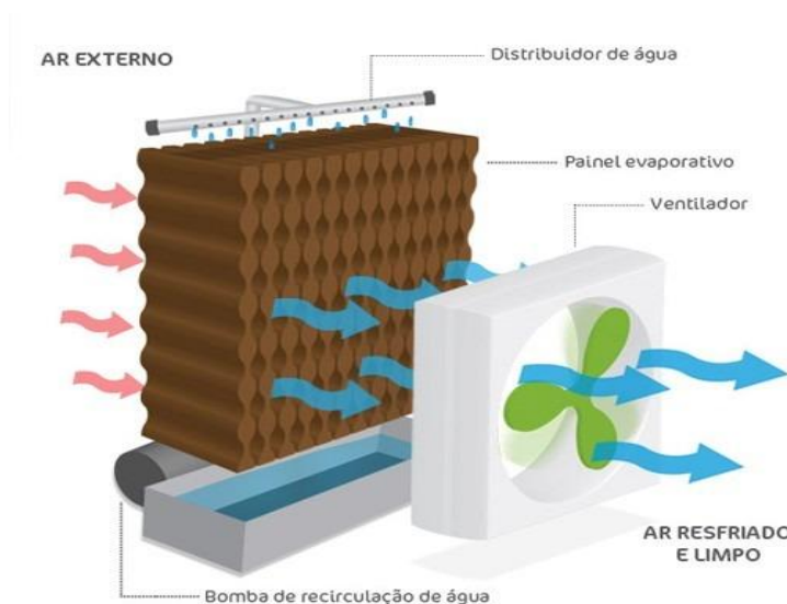
Figura 1 – Funcionamento ilustrativo do climatizador evaporativo.
